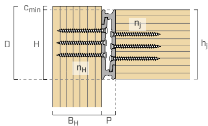
trave secondaria
