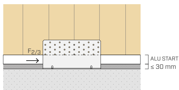
PRZYKŁAD INSTALACJI Z UŻYCIEM TITAN TCN240
