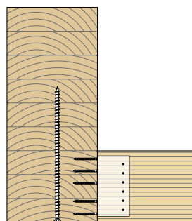
presjek
