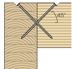
Aufriss
