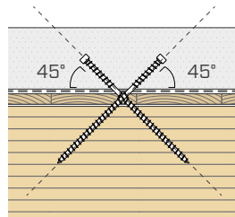
Montare încrucișată la 45° cu sau fără folie fonoizolantă.
